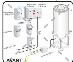
Branchements standard d'un chauffe-eau électrique HC/HP
