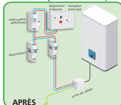
Installation du chauffe-eau Plat branchement permanent uniquement
